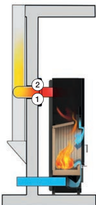
Kaminofen
